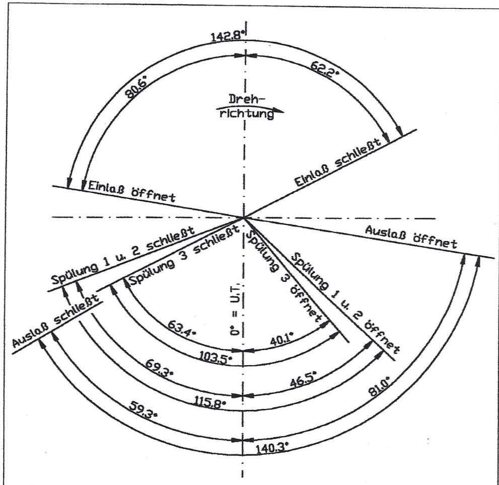
Steuerdiagramm der Type 250 MCH mit dem größten Einlaßsteuerwinkel aller Typen.
